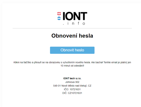
Obr. 9: Verifikační e-mail
